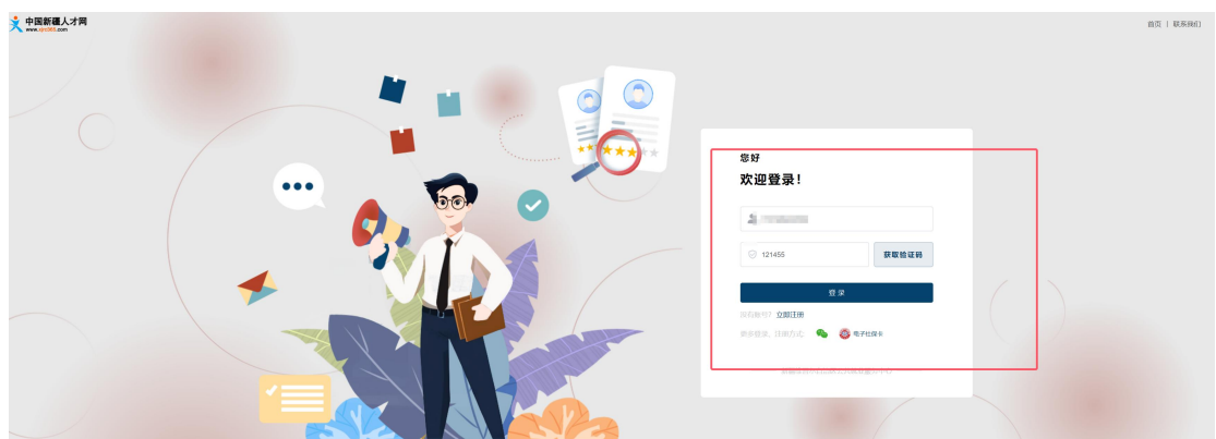
图 6 登录界面
